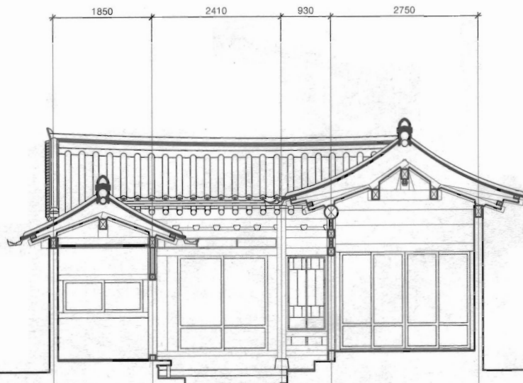
A-A'단면도
