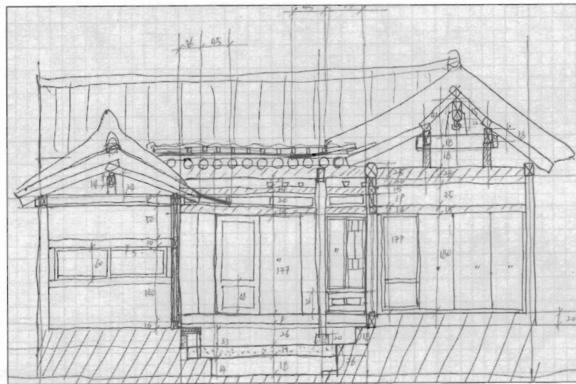
실측도면(단면)
