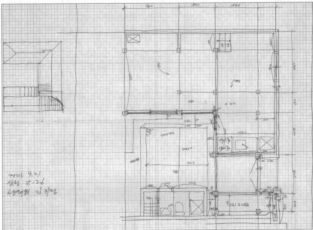
실측도면(평면)
